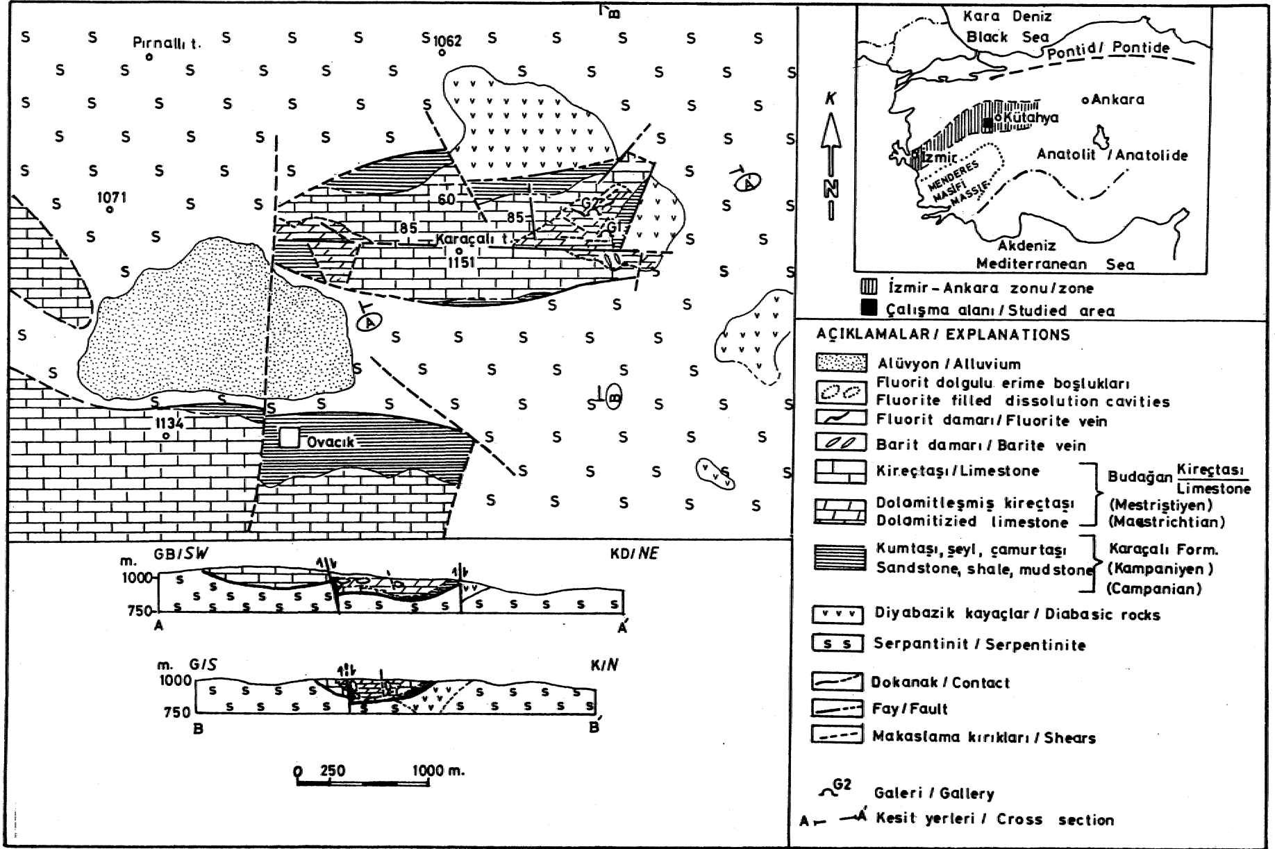
Şekil 1 Ovacık yöresi jeolojî haritası
