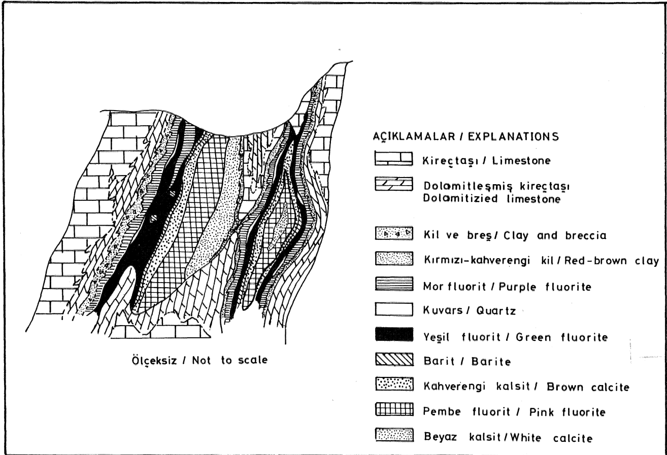
Şekil 3 Erime boşluklarında ve damarlarda gelişen simetric ve asimetric bantlı dolgular
